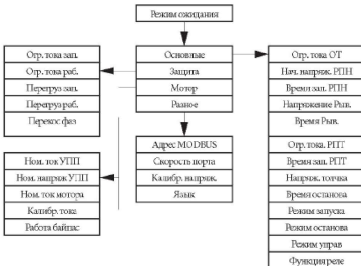
Рис. 8-1 Архитектура меню.
