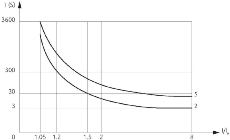
Рис. 9-1 Характеристика защиты двигателя от перегрузки.
